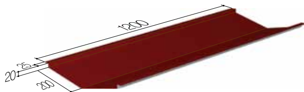
Укрытие ендовы ROMAN
