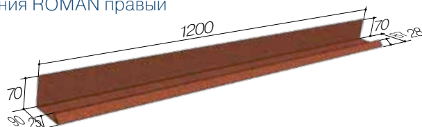
Элемент примыкания ROMAN правый
